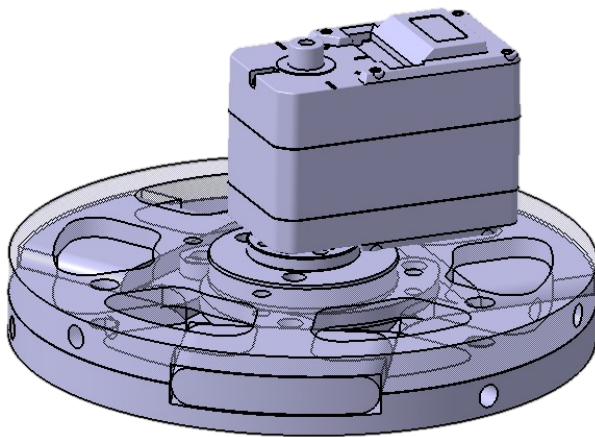
FIGURE 4.8 – Système d'aérofrein d'SP-02 sur CA-TIA
