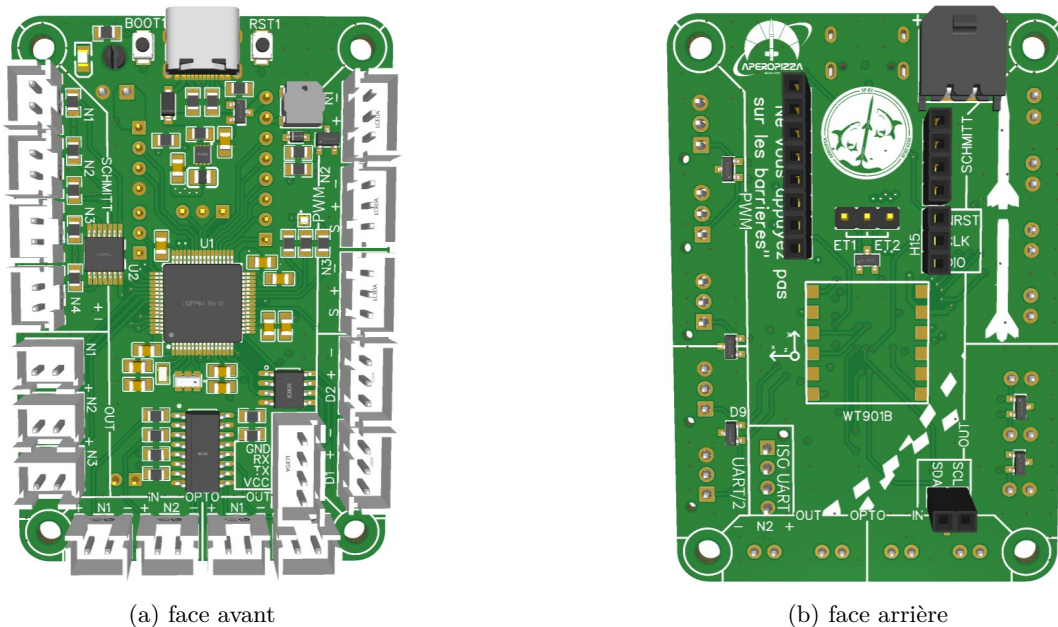
FIGURE 5.6 – Rendu 3D de la carte séquenceur
