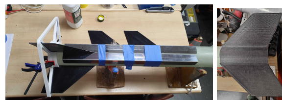
(a) Collage surfacique des ailerons (b) Renfort
