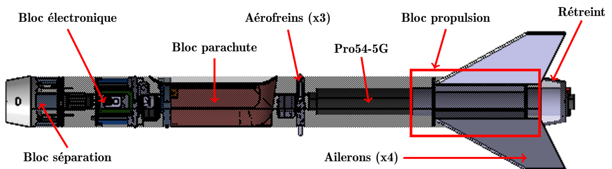
FIGURE 1.2 – Vue du premier étage sur CATIA
