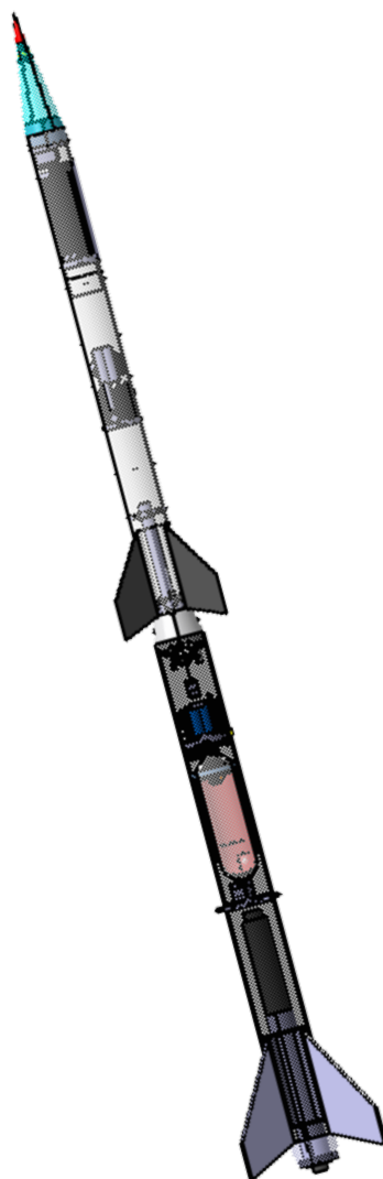
FIGURE 1.4 – Vue d’ensemble de la fusée SP-02 sur CATIA
