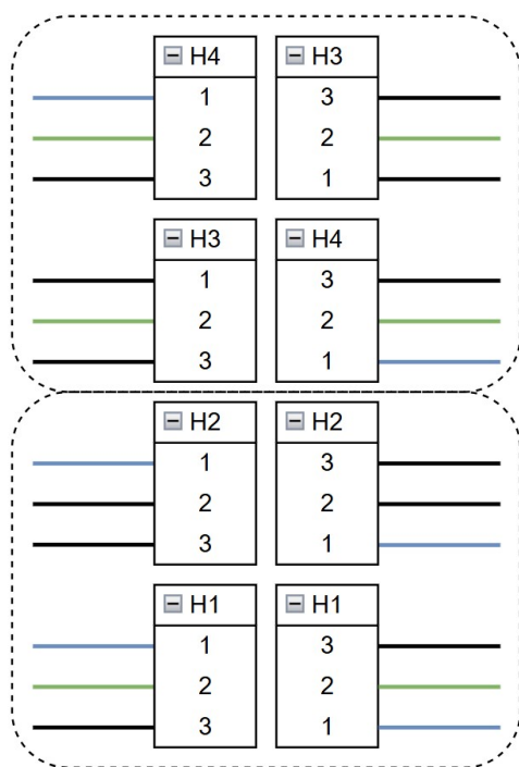
FIGURE 5.3 – Schéma de la connexion inter-étage
