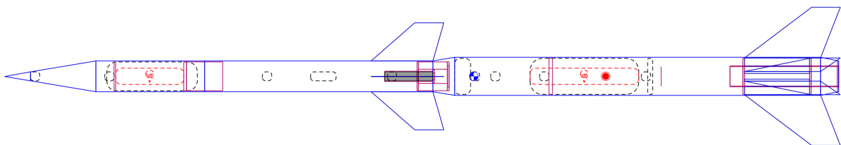
FIGURE 3.1 – Modélisation de la fusée SP-02 dans OpenRocket
