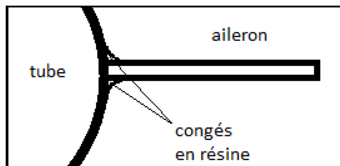
FIGURE 4.3 – Procédé de collage ailerons/structure avec congés en résine
