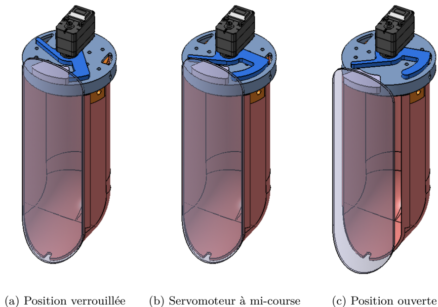
FIGURE 4.12 – Bloc parachute du premier étage sur CATIA
