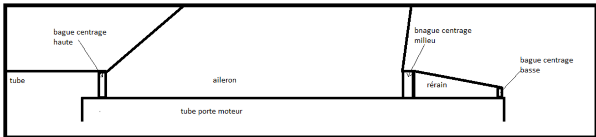
FIGURE 4.2 – Procédé de collage ailerons/tube porte-moteur
