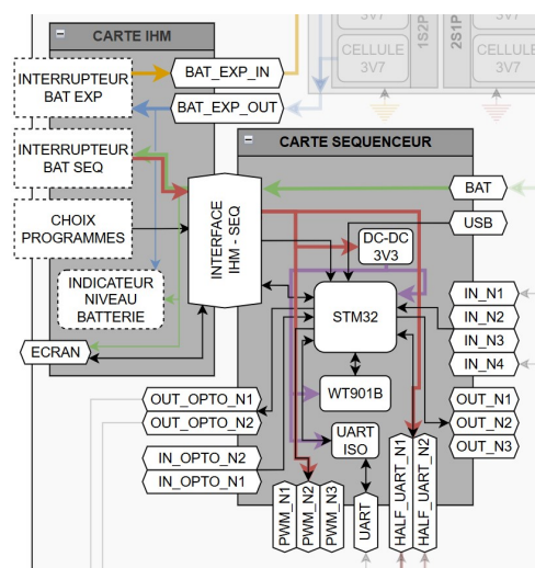
FIGURE 5.7 – Zoom sur le séquenceur et interface
