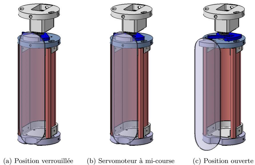
FIGURE 4.20 – Bloc parachute du second étage sur CATIA
