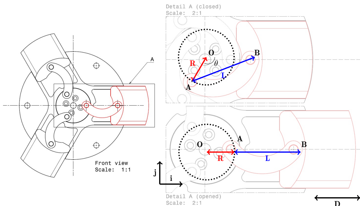
FIGURE 4.11 – Schéma de la cinématique des aérofreins
