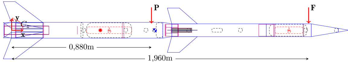
FIGURE 4.1 – Schéma de calcul du couple exercé au niveau de la base du premier étage
