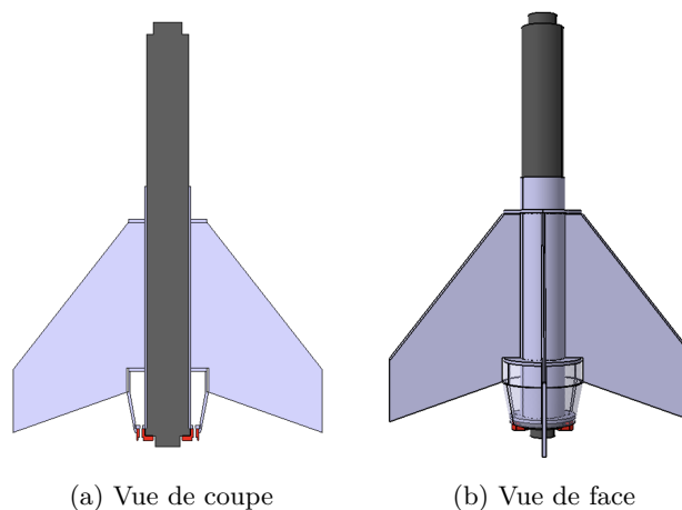
FIGURE 4.6 – CAO du bloc propu du preier étage(Pro-54 6G)
