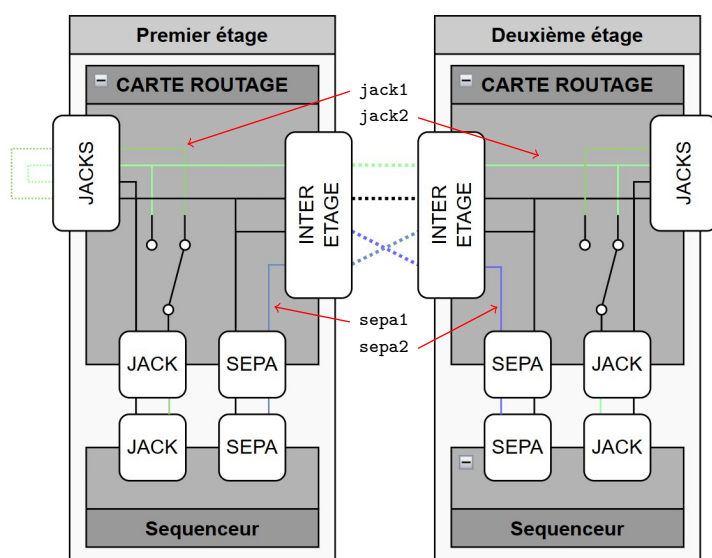
FIGURE 5.2 – Système de détection du décollage et de la séparation inter-étage
